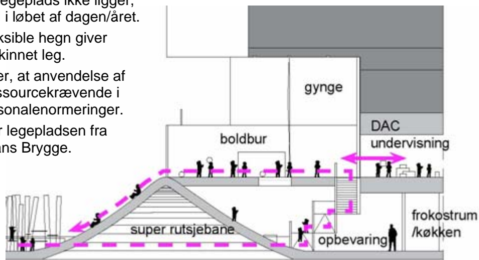
Tegningen viser et snit i legeplads for de mindste børn. Der er indarbejdet rum til opbevaring af institutionernes legeting, køkken og toilet.
